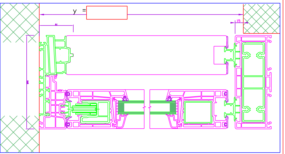
COUPE VERTICALE
